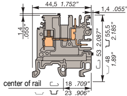
MA 2,5/5.CPE...
